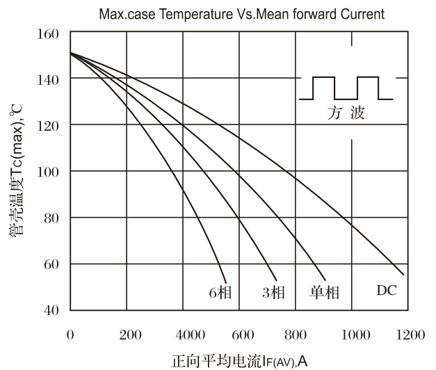
Fig.6 管壳温度与正向平均电流关系曲线
